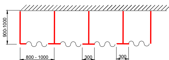
Duschtrennwände mit Frontteilen
