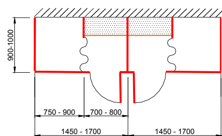
Duschkabine mit Umkleidebereich, Tür nach außen
